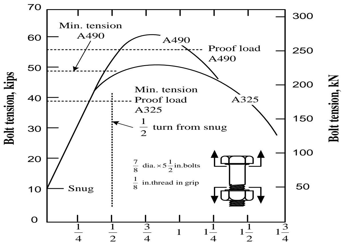
圖 1 螺栓之軸拉力-軸向變形關係曲線
